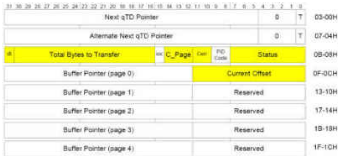
Gambar 4.6 Struktur data Queue Head.
